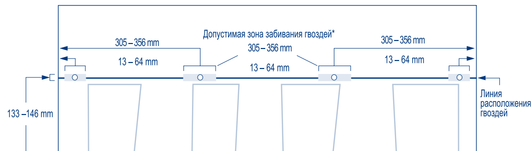
Схема крепления четырьмя гвоздями
